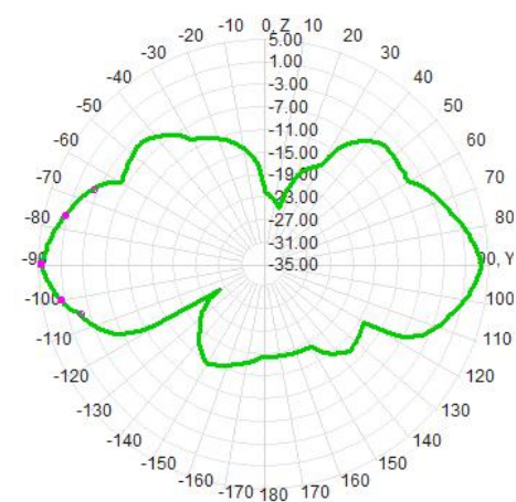
E2面-PHI=90
