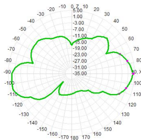
E1面-PHI=0
