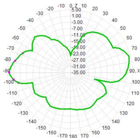
E1面-PHI=0
