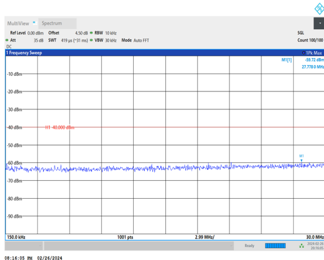
Band30-10MHz-QPSK-27710-1RB#0-Range2:0.15~30MHz
