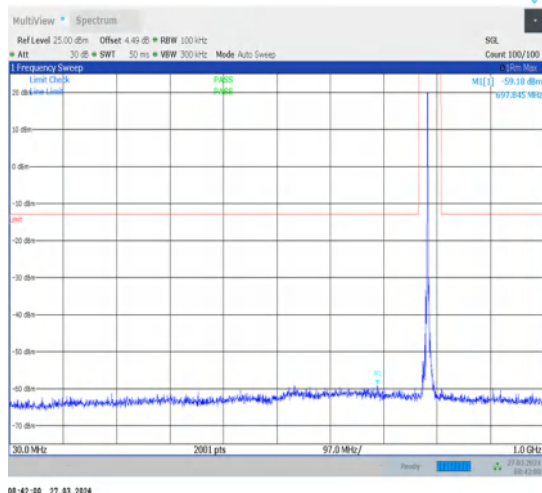
1-N14-15-10-L-1-DFT-PI2BPSK-Inner_1RB_Left- 1@1-30-1000-Ant1-697.85--59.18--13-PASS
