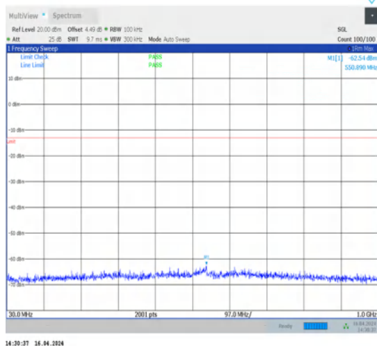
1-N78-3700-3800-N78-3700-380030-100-L-1-DFT-PI2BPSK-Inner_1RB_Left-1@1-30-1000-Ant1-529.55--62.54--13-PASS
