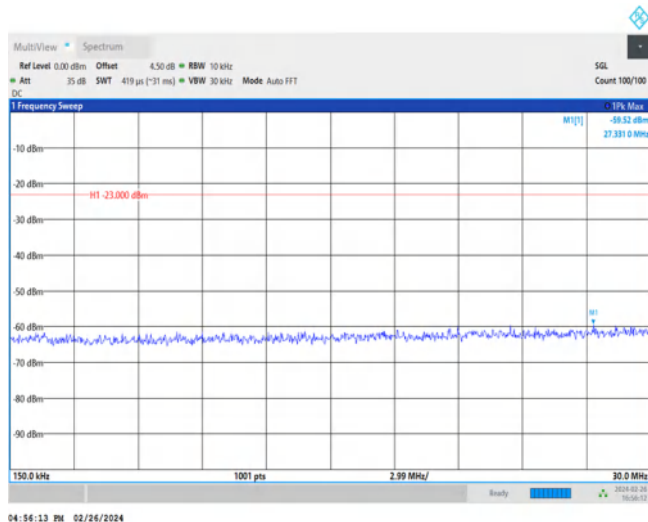
Band25-20MHz-QPSK-26140-1RB#0-Range2:0.15~30MHz
