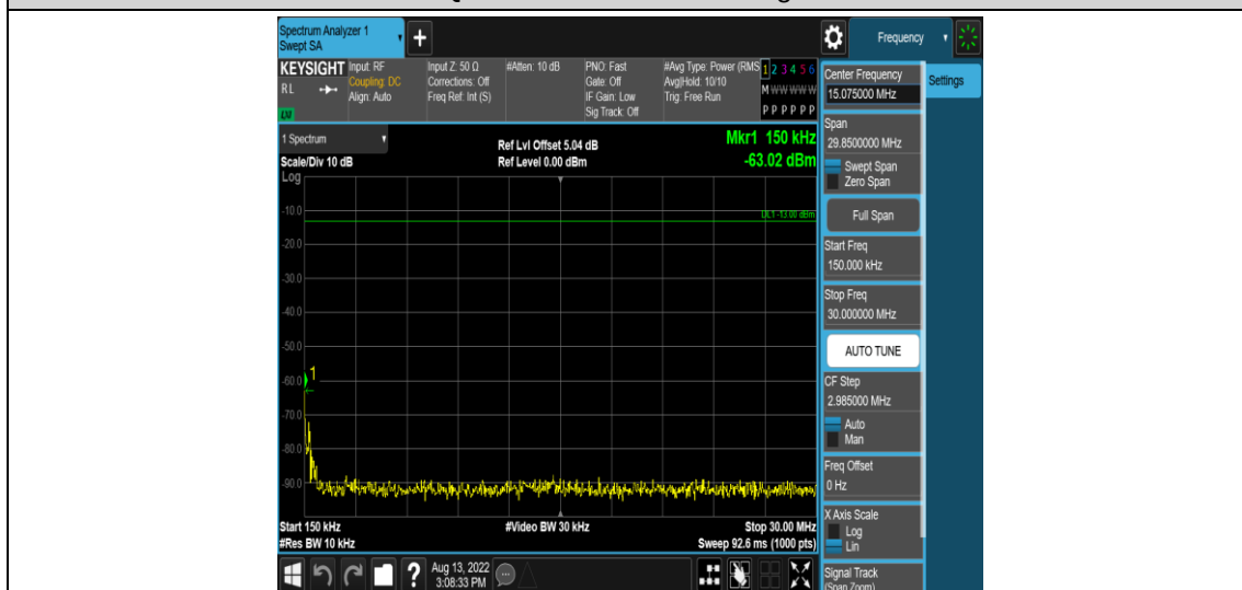
Band12-1.4MHz-QPSK-23095-1RB#0-Range2:0.15~30MHz
