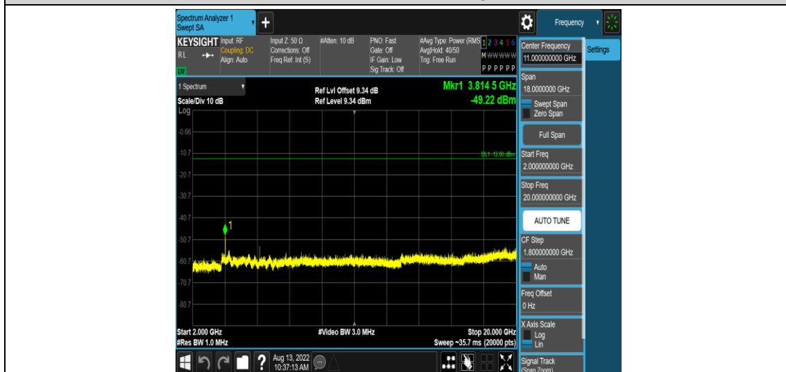
Band2-3MHz-QPSK-19185-1RB#0-Range5:2000~20000MHz
