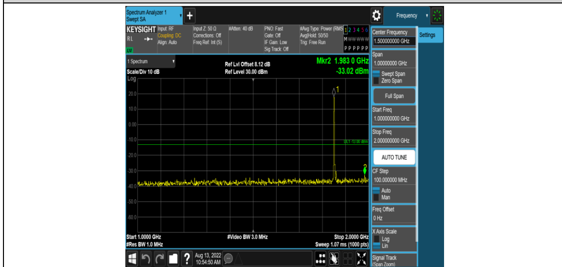
Band2-5MHz-QPSK-18625-1RB#0-Range4:1000~2000MHz
