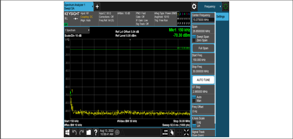
Band2-5MHz-QPSK-19175-1RB#0-Range2:0.15~30MHz
