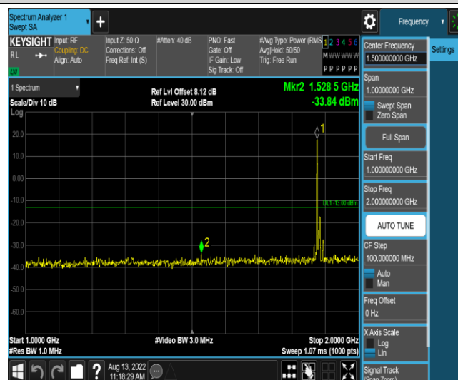
Band2-10MHz-QPSK-18900-1RB#0-Range4:1000~2000MHz
