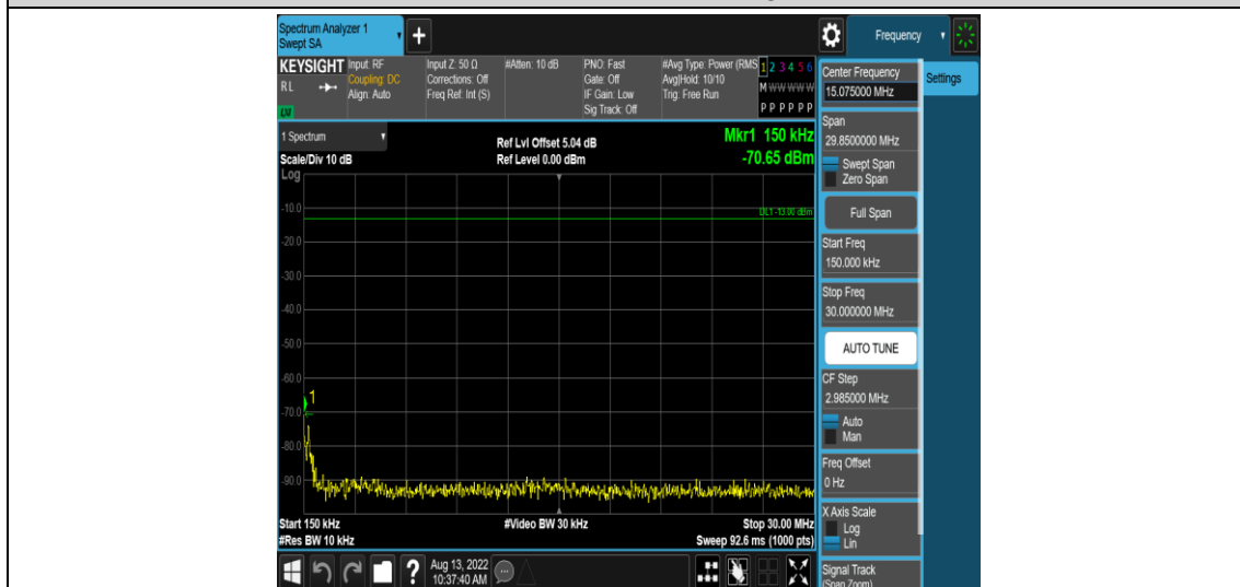
Band2-3MHz-16QAM-19185-1RB#0-Range2:0.15~30MHz
