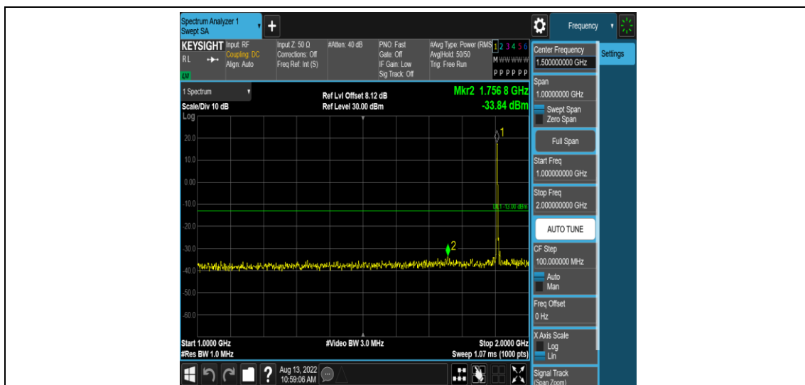
Band2-5MHz-QPSK-19175-1RB#0-Range4:1000~2000MHz
