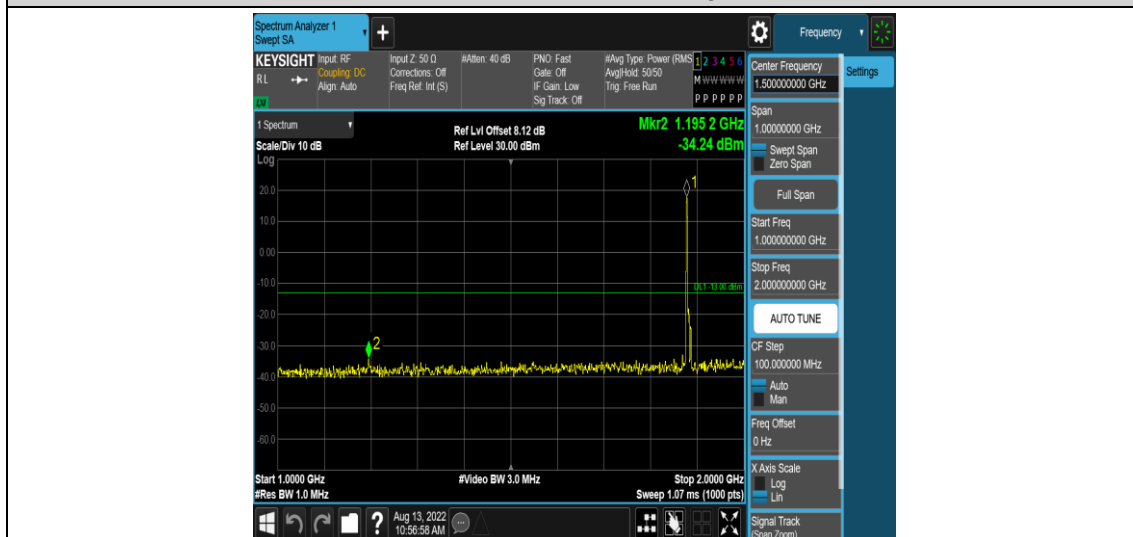
Band2-5MHz-QPSK-18900-1RB#0-Range4:1000~2000MHz
