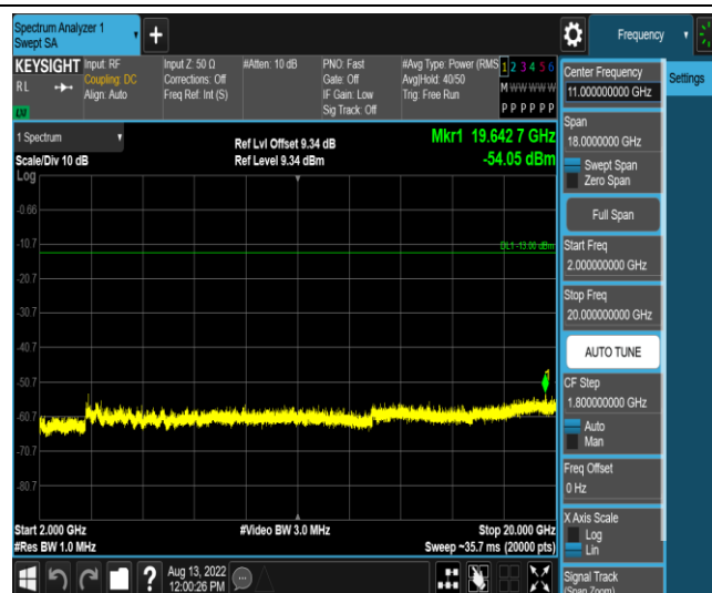
Band2-20MHz-QPSK-18700-1RB#0-Range5:2000~20000MHz
