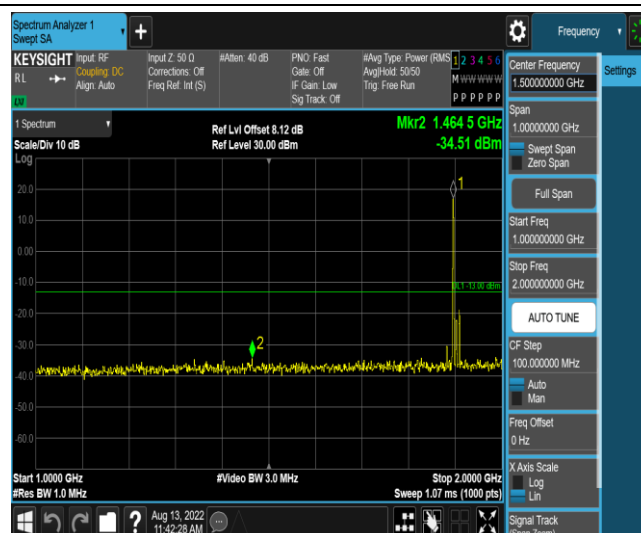
Band2-15MHz-QPSK-19125-1RB#0-Range4:1000~2000MHz
