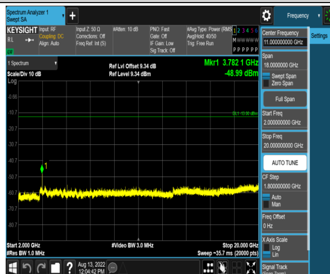
Band2-20MHz-QPSK-19100-1RB#0-Range5:2000~20000MHz
