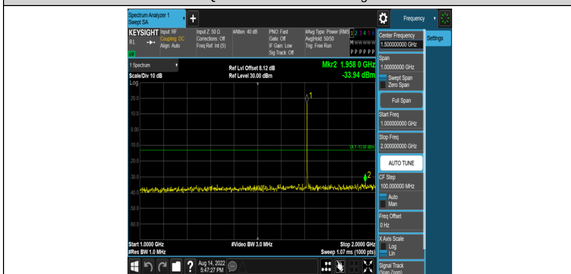
Band4-1.4MHz-QPSK-19957-1RB#0-Range4:1000~2000MHz
