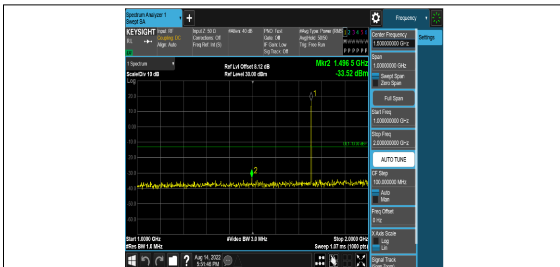
Band4-1.4MHz-QPSK-20393-1RB#0-Range4:1000~2000MHz
