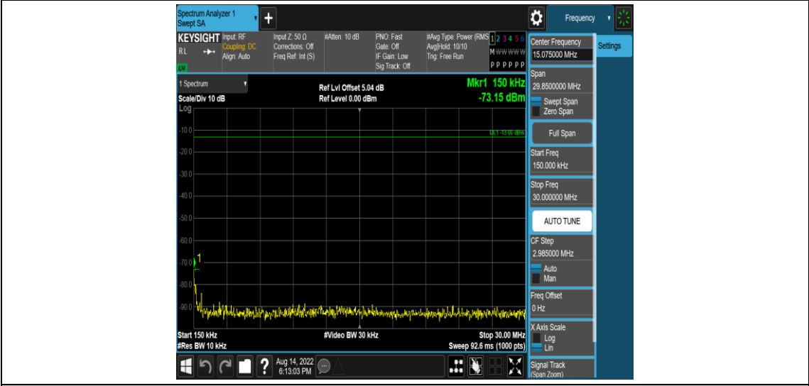
Band4-3MHz-QPSK-20385-1RB#0-Range2:0.15~30MHz
