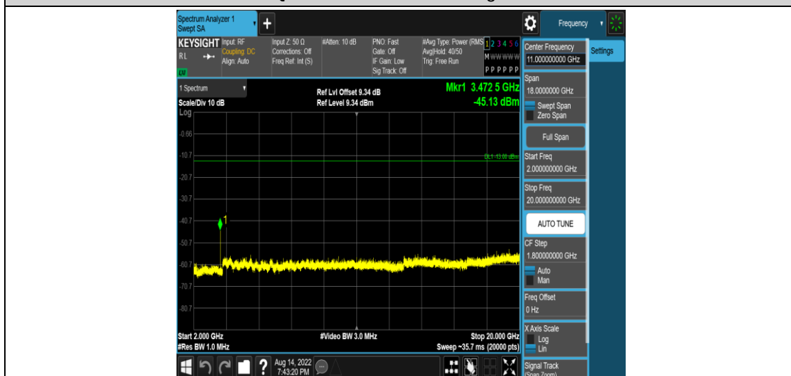
Band4-20MHz-QPSK-20300-1RB#0-Range5:2000~20000MHz
