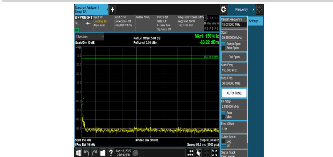
Band5-3MHz-QPSK-20525-1RB#0-Range2:0.15~30MHz
