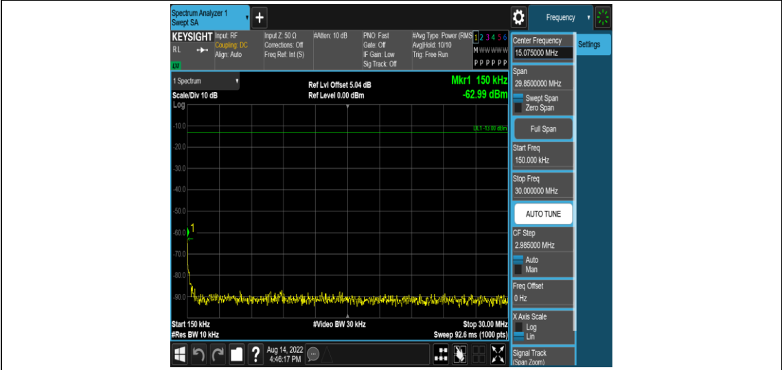
Band71-10MHz-QPSK-133297-1RB#0-Range2:0.15~30MHz
