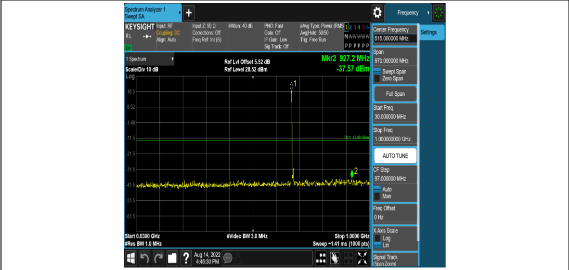
Band71-10MHz-QPSK-133297-1RB#0-Range3:30~1000MHz
