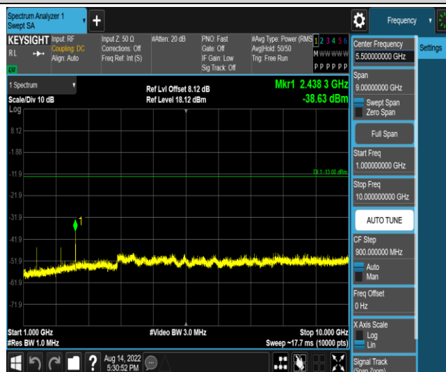
Band71-20MHz-QPSK-133372-1RB#0-Range4:1000~10000MHz
