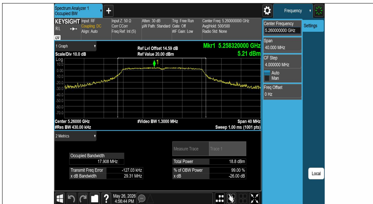
11A-Ant1-5260
