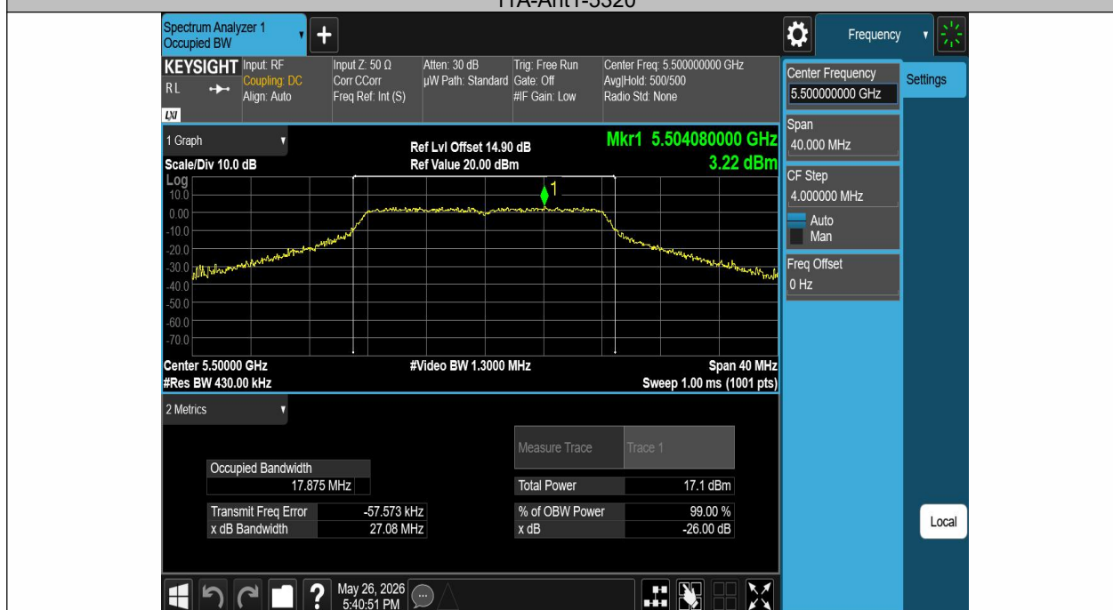
11A-Ant1-5500
