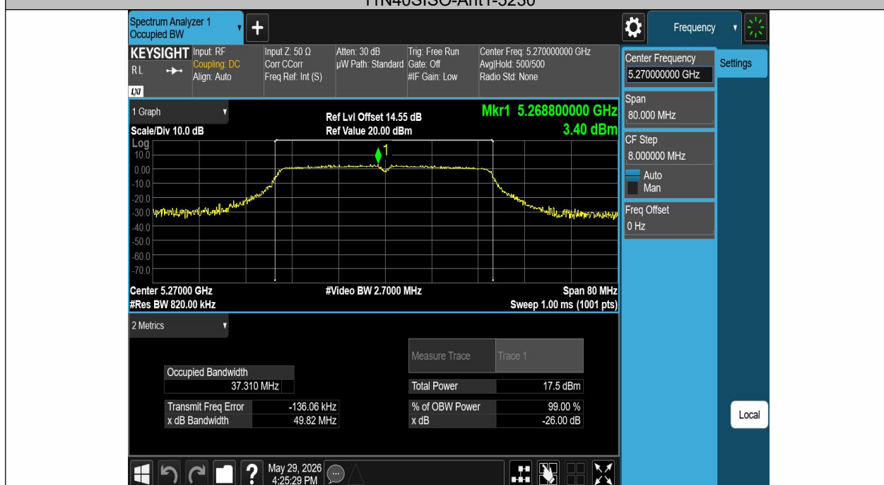
11N40SISO-Ant1-5270
