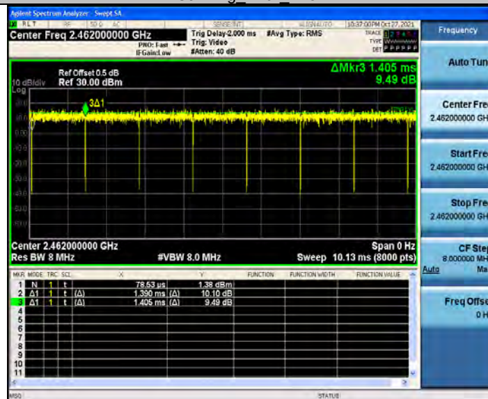
802.11g Ant2 2462
