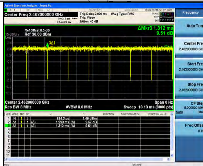
802.11n(HT20) Ant2 2462
