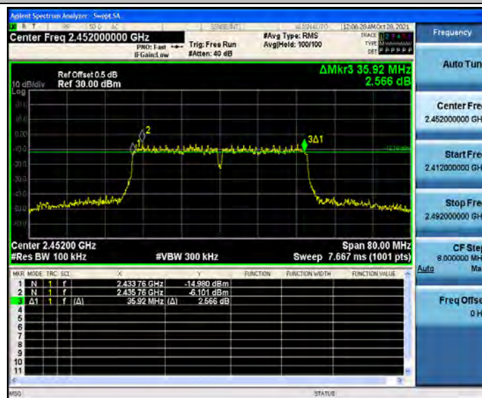
802.11n(HT40)_Ant2_2452
