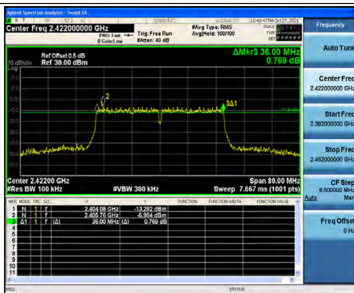
802.11n(HT40)_Ant2_2422
