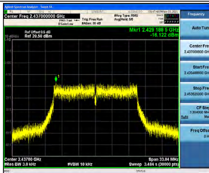
802.11g_Ant2_2437
