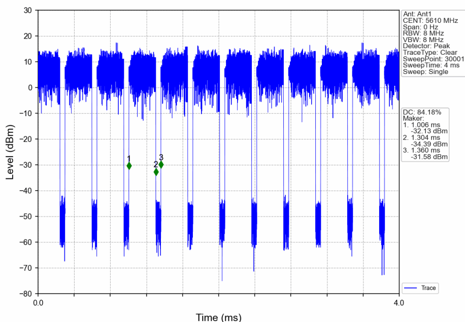
802.11ax(HEW80)_HCH_5610MHz_RU996_Left_Ant1_NTNV
