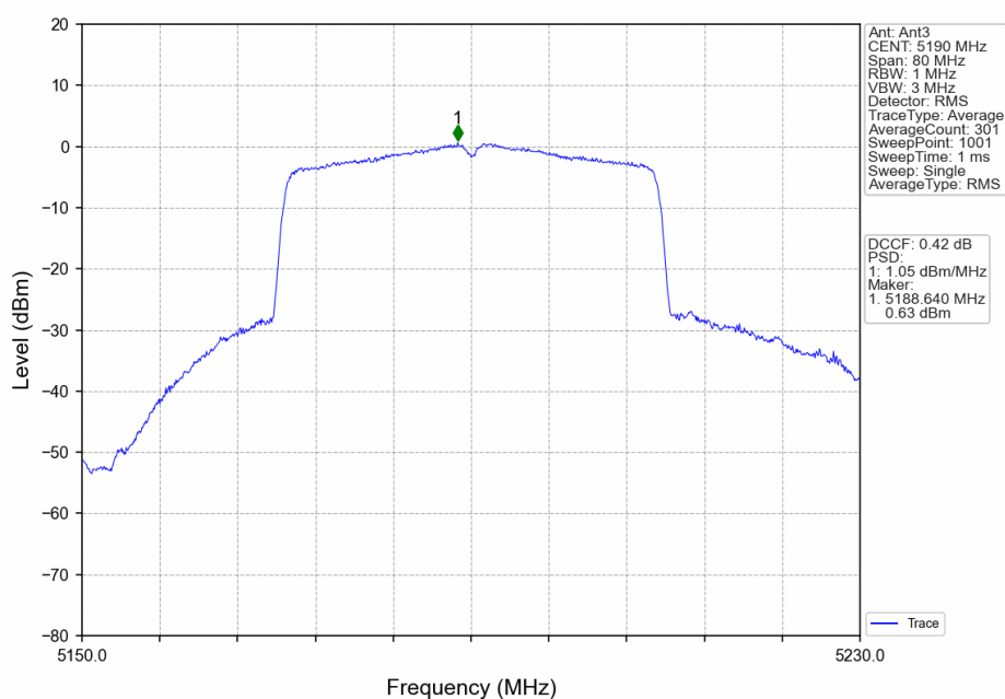
802.11ax(HEW40)_LCH_5190MHz_RU484_Left_Ant3_NTNV
