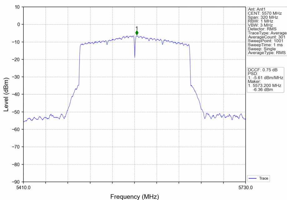
802.11ax(HEW160)_MCH_5570MHz_2xRU996_Left_Ant1_NTNV
