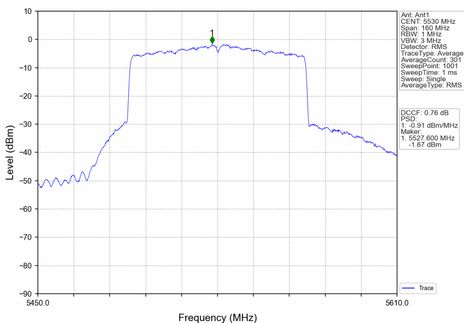
802.11ax(HEW80)_LCH_5530MHz_RU996_Left_Ant1_NTNV
