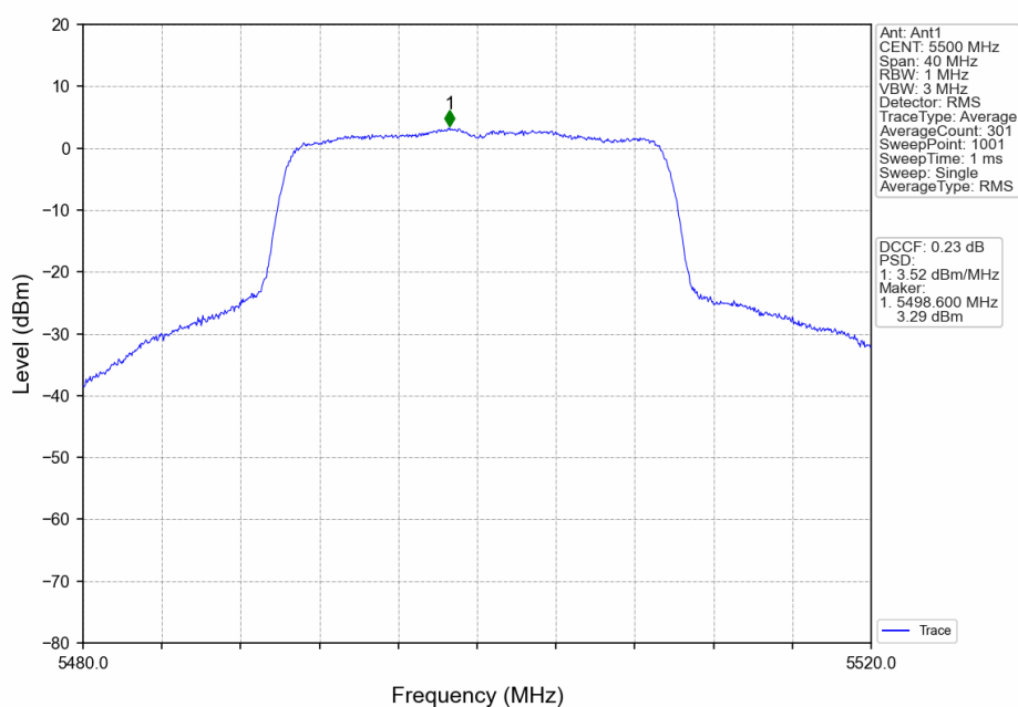
802.11ax(HEW20)_LCH_5500MHz_RU242_Left_Ant1_NTNV
