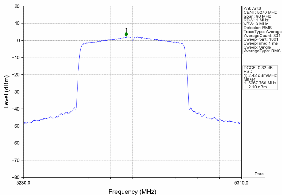
802.11ax(HEW40)_LCH_5270MHz_RU484_Left_Ant3_NTNV
