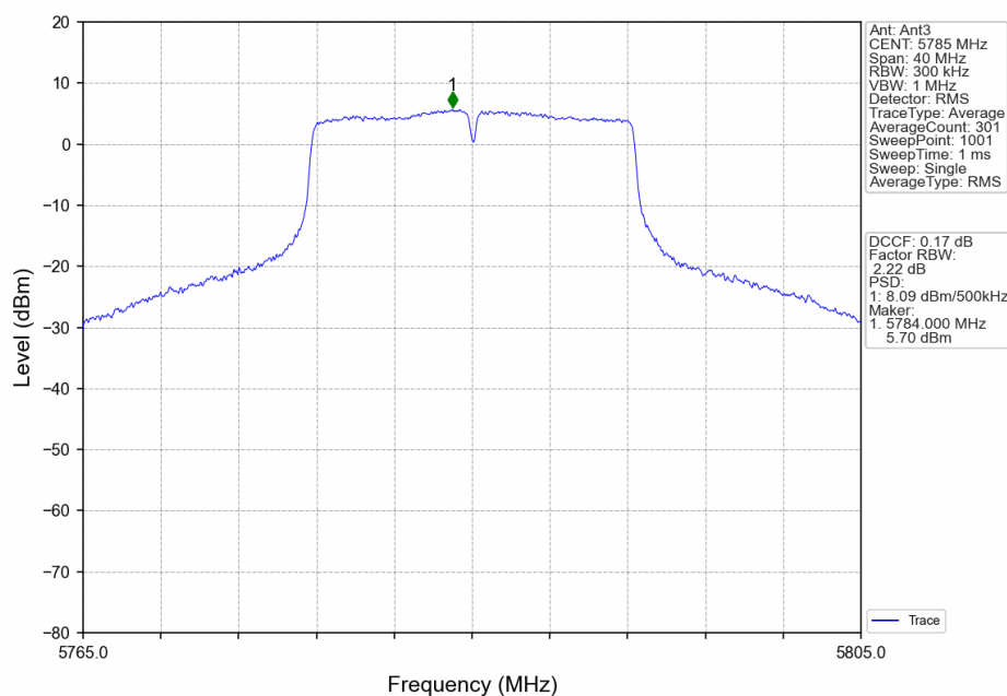
802.11a_MCH_5785MHz_Ant3_NTNV
