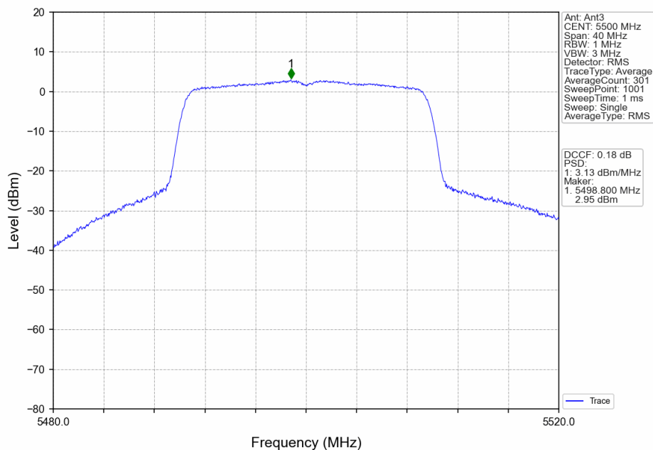
802.11ax(HEW20)_LCH_5500MHz_RU242_Left_Ant3_NTNV
