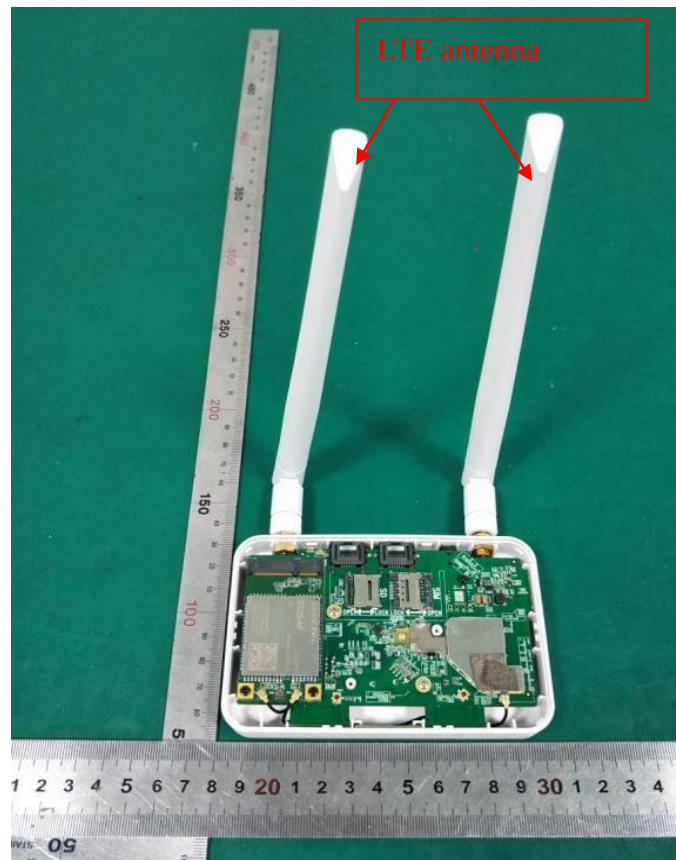
EUT-8
