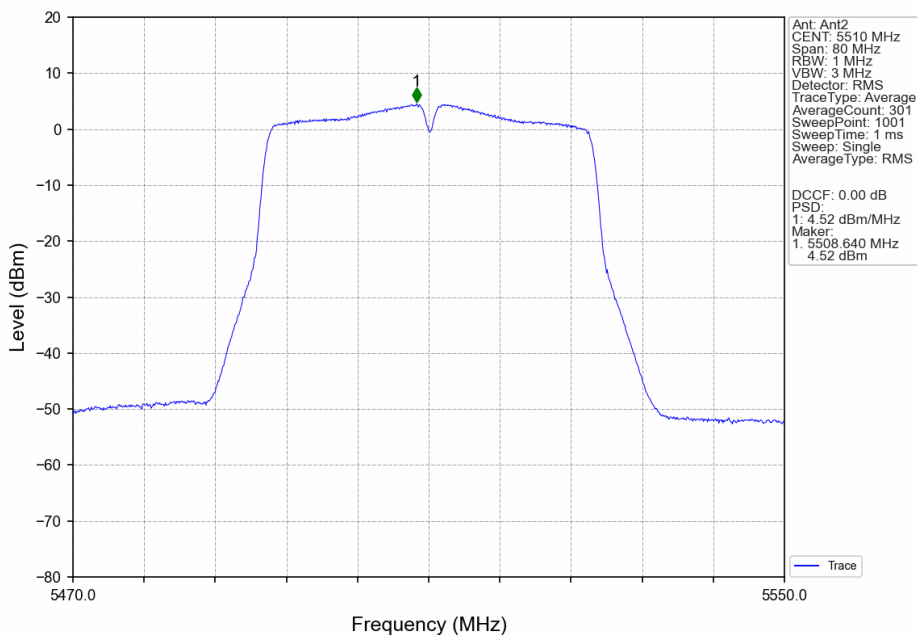
802.11n(HT40)_LCH_5510MHz_Ant2_NTNV
