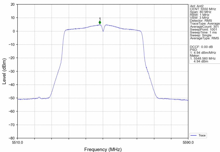
802.11n(HT40)_MCH_5550MHz_MIMO_NTNV
