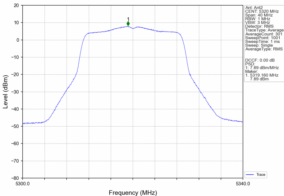
802.11n(HT20)_HCH_5320MHz_Ant2_NTNV
