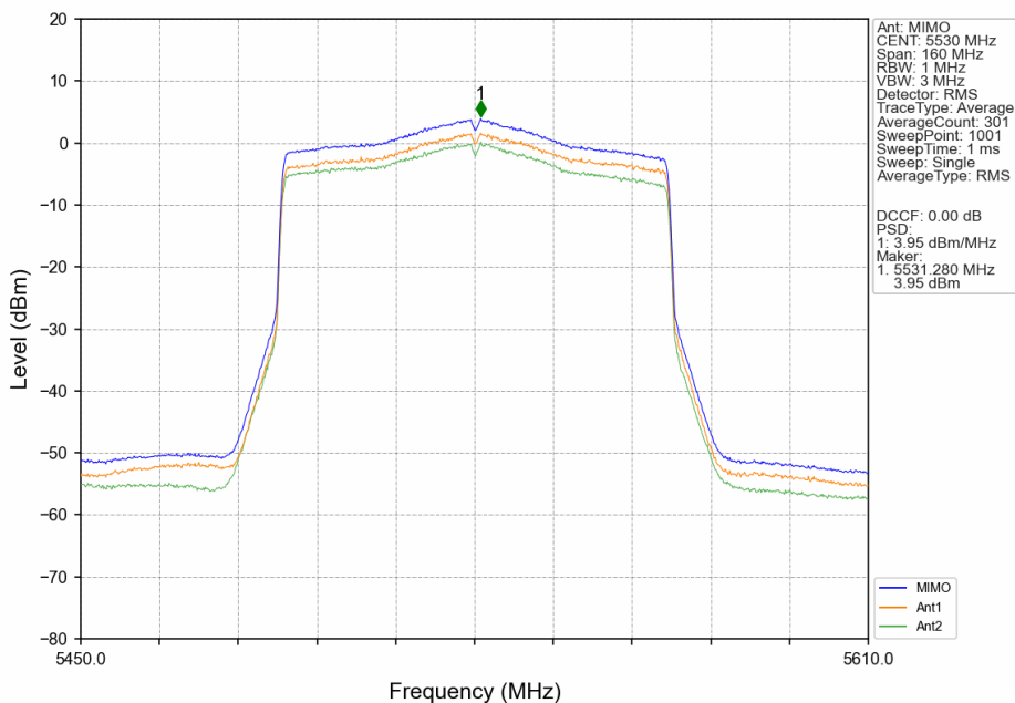
802.11ax(HEW80)_LCH_5530MHz_RU996_Left_MIMO_NTNV
