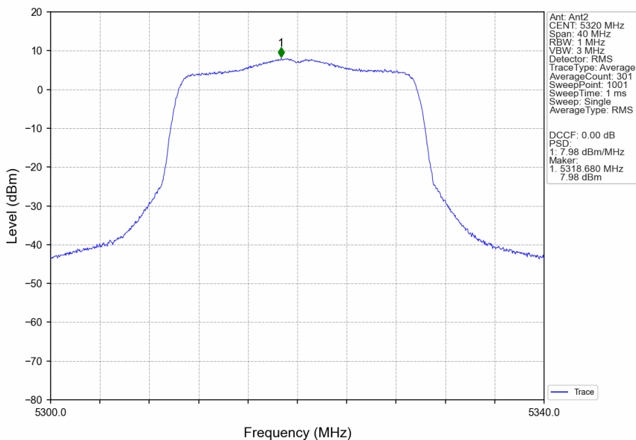
802.11ax(HEW20)_HCH_5320MHz_RU242_Left_Ant2_NTNV
