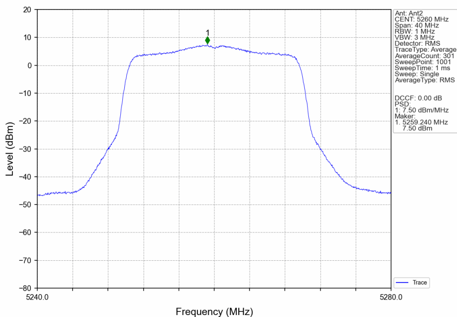
802.11ax(HEW20)_LCH_5260MHz_RU242_Left_Ant2_NTNV
