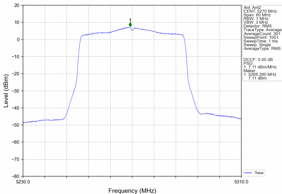
802.11ax(HEW40)_LCH_5270MHz_RU484_Left_Ant2_NTNV
