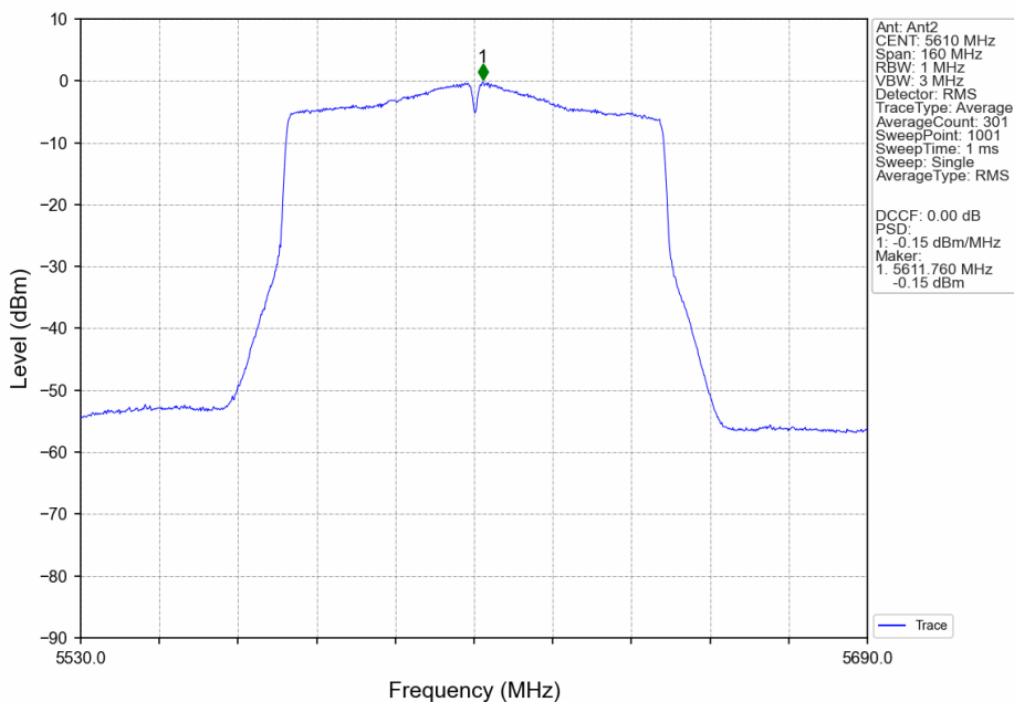
802.11ac(VHT80)_HCH_5610MHz_Ant2_NTNV
