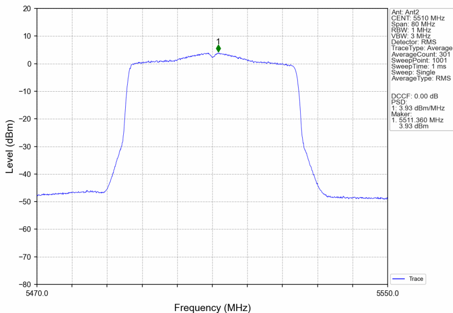
802.11ax(HEW40)_LCH_5510MHz_RU484_Left_Ant2_NTNV
