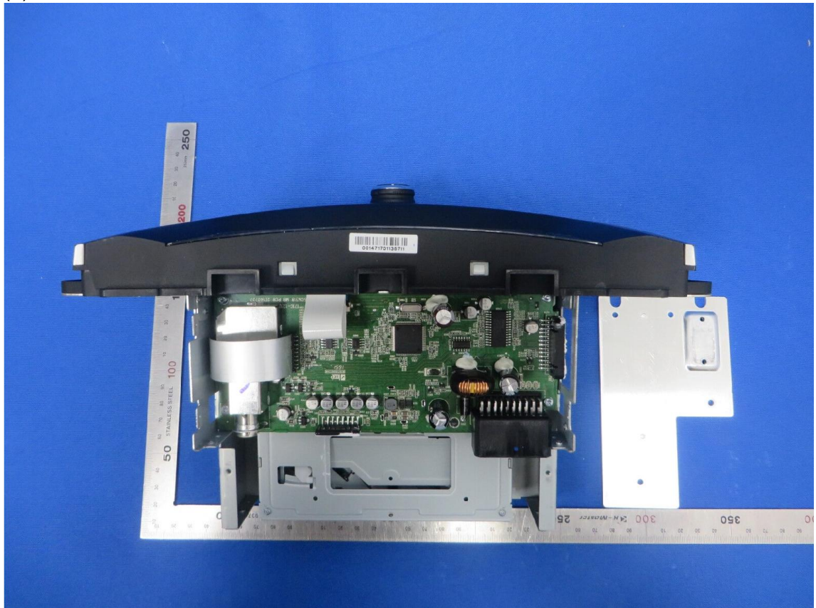
(4) EUT Photo
