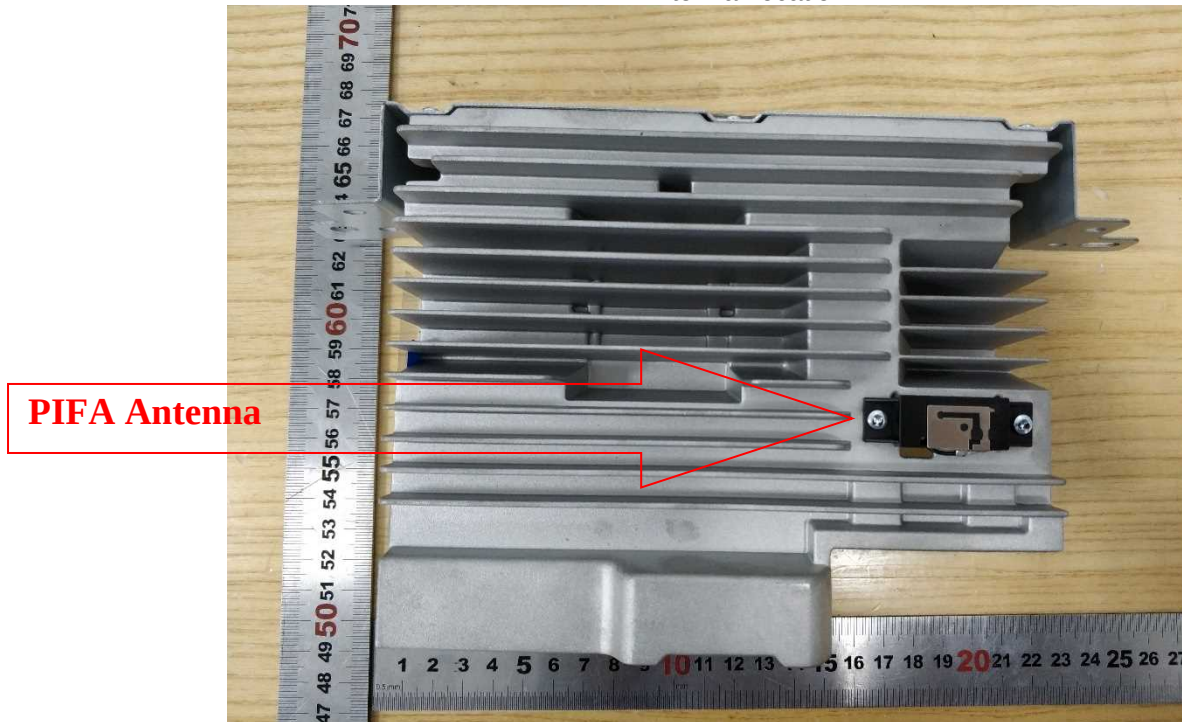
PIFA Antenna
