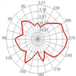
5200.000MHz E1
