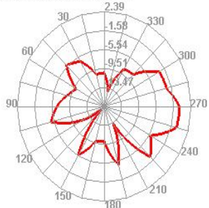
5550.000MHz E1
