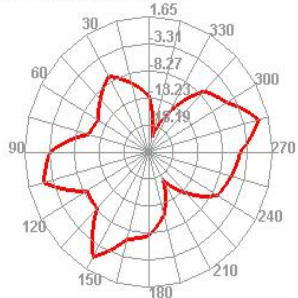
6000.000MHz E1
