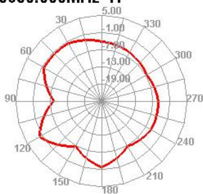
5650.000MHz H
