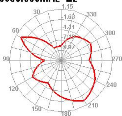
5650.000MHz E2
