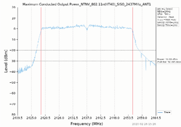
802.11n(HT40) 2437MHz_SISO_ANT1
