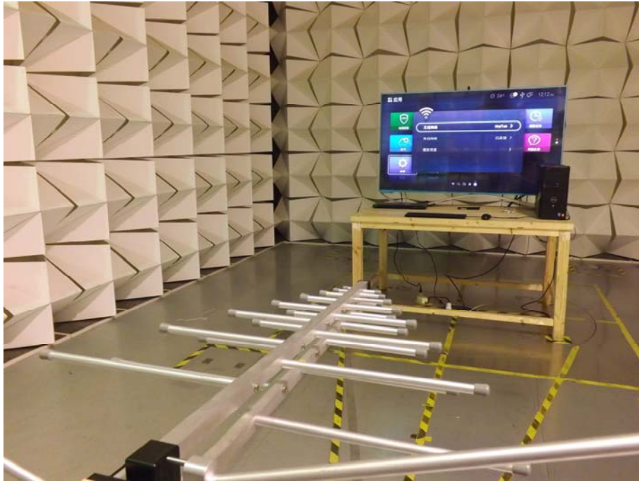
For 30MHz-1000MHz
