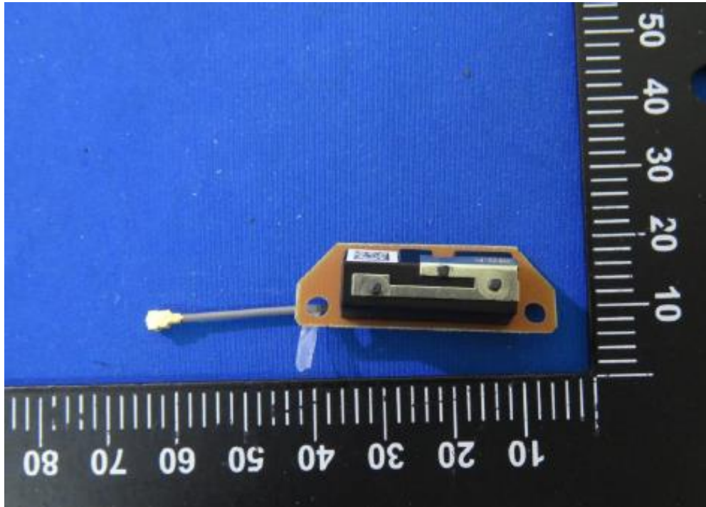
PIFA Antenna (SMARTEQ 4211613980)
