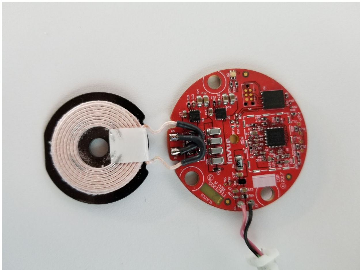
PCBA TOP
