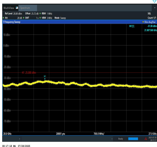
Band7-20MHz-QPSK-20850-100RB#0-20000~2 7000-PASS
