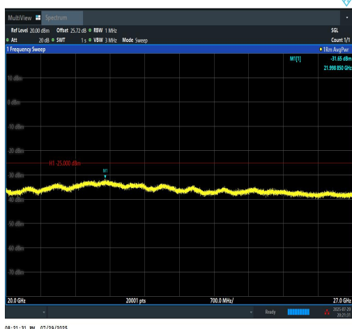
Band7-20MHz-QPSK-21100-1RB#0-20000~270-00-PASS
