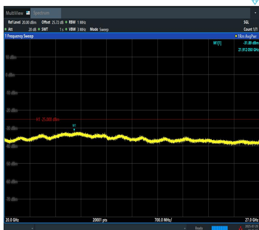
Band7-20MHz-QPSK-21350-100RB#0-20000~2 7000-PASS
