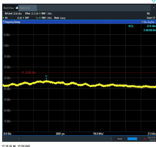
Band7-15MHz-QPSK-20825-1RB#0-20000~270-00-PASS
