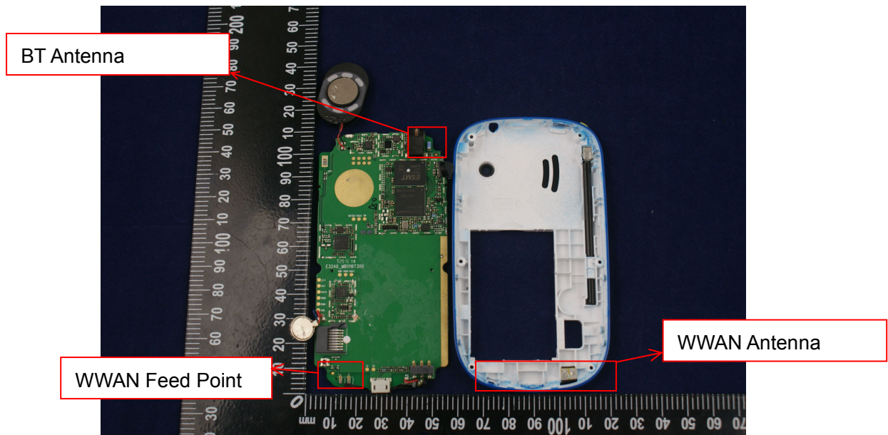
EUT Photo 7
