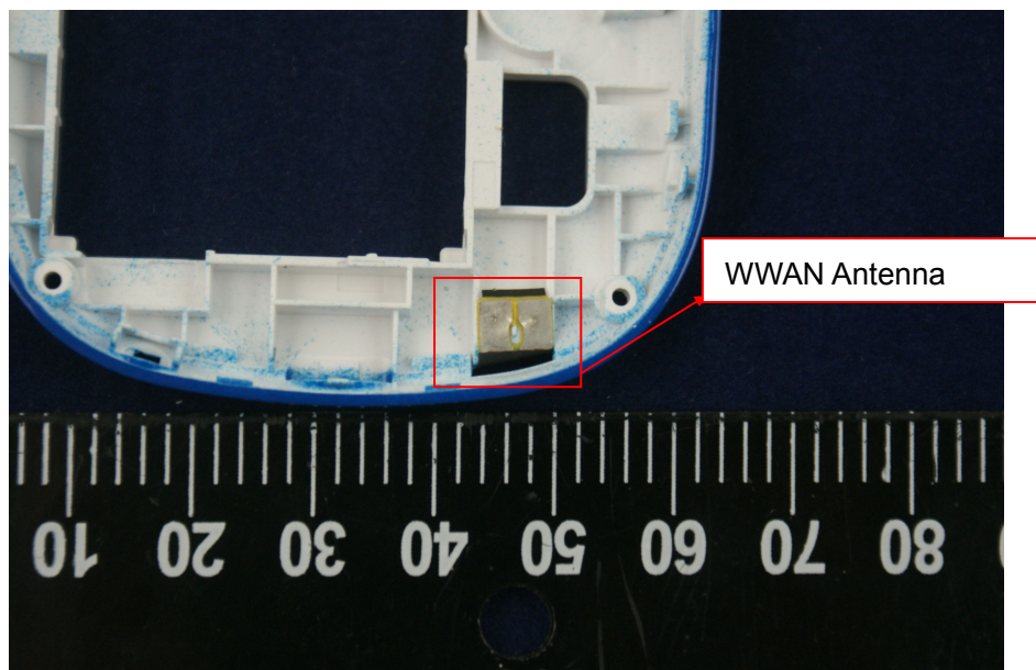
EUT Photo 8
