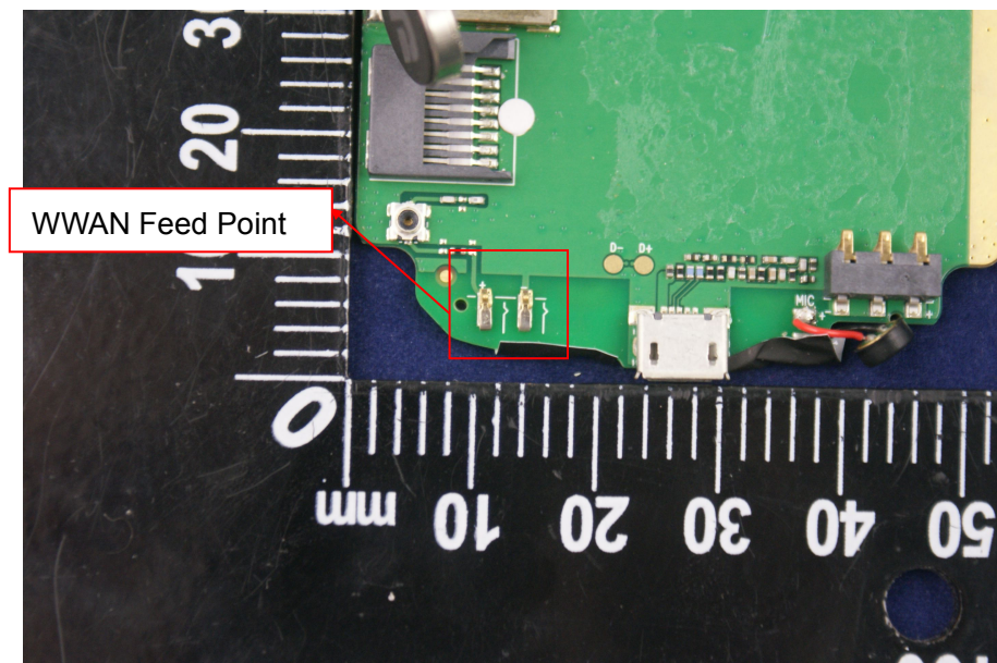
EUT Photo 10
