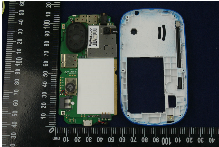
EUT Photo 4
