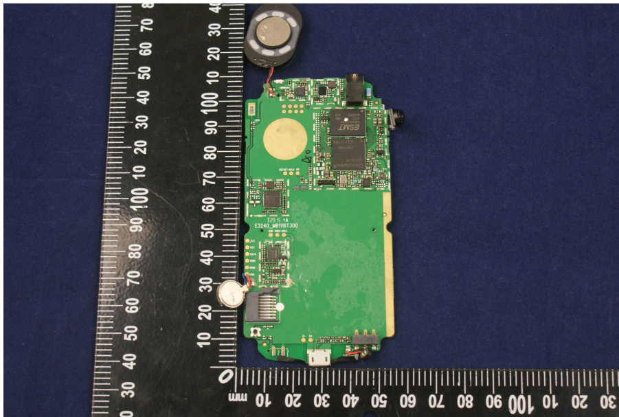
EUT Photo 6
