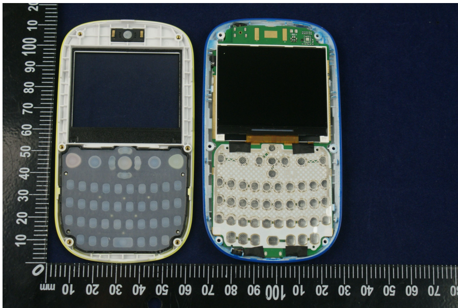
EUT Photo 2
