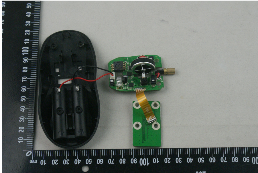
EUT Photo 3
