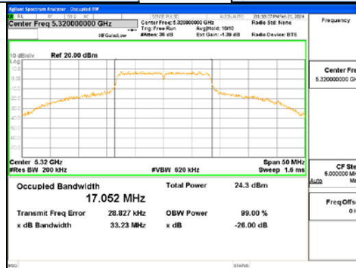
802.11a_UNII 2A
