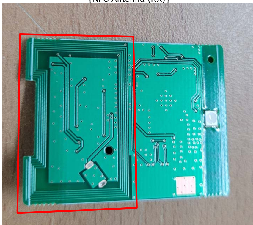
{NFC Antenna (RX)}
