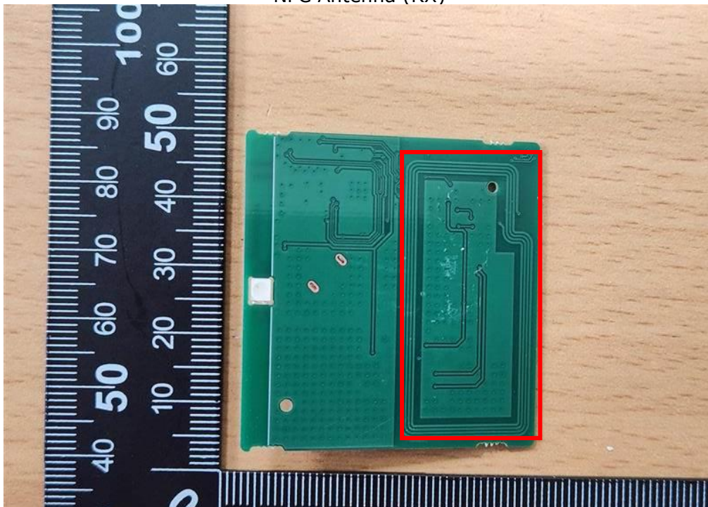
NFC Antenna (RX)
