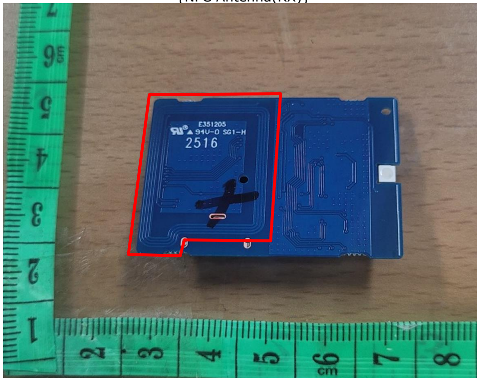
{NFC Antenna(RX)}
