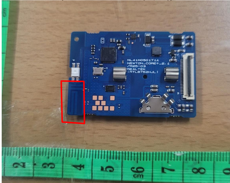
{NFC Antenna(RX)}
