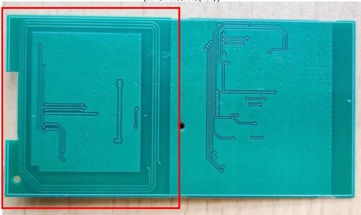
{NFC Antenna(RX)}
