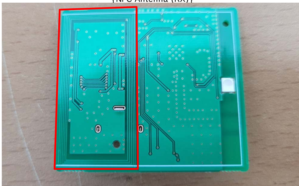
{ NFC Antenna (RX) }
