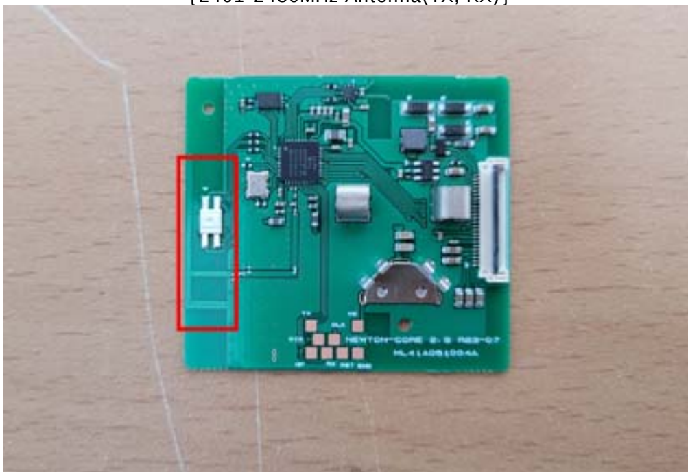
{ 2401-2480MHz Antenna(TX, RX) }
