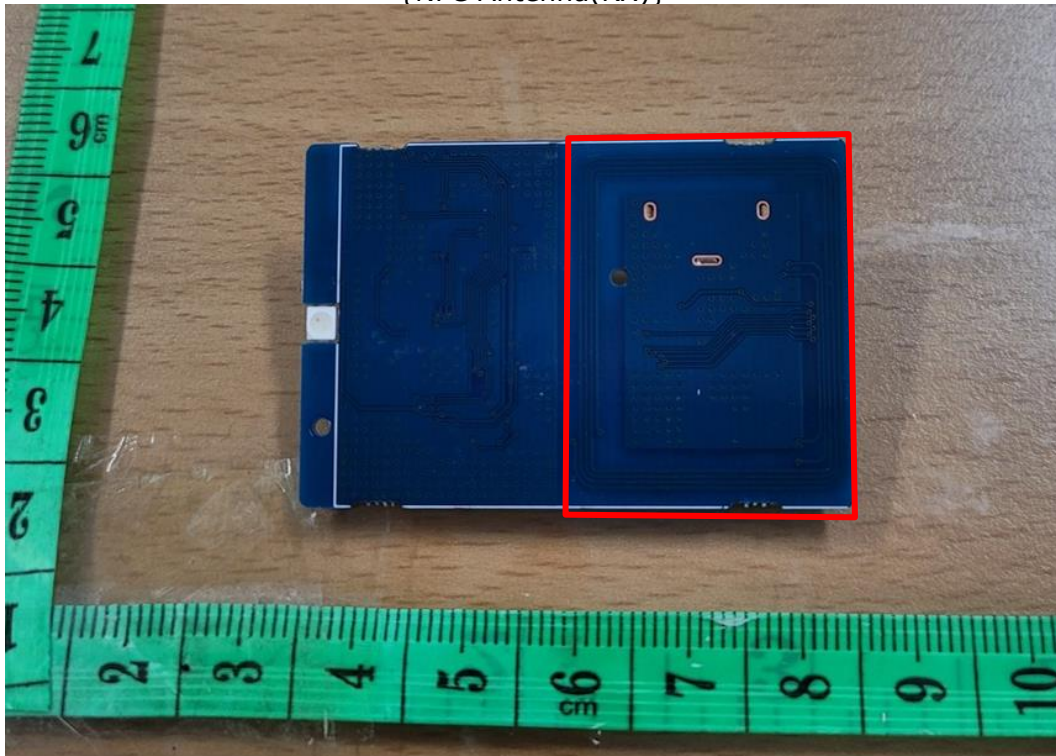
{NFC Antenna(RX)}
