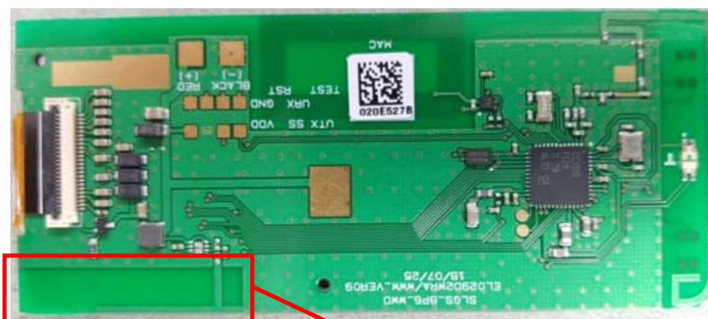
Wake up Antenna(RX)
