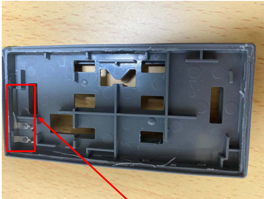
Antenna(TX, RX)
