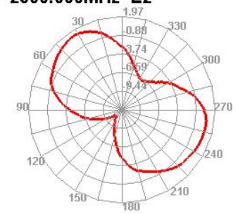
2500.000MHz E2
