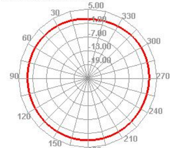
2450.000MHz H
