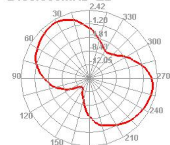
2450.000MHz E2
