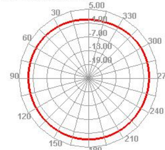
2500.000MHz H
