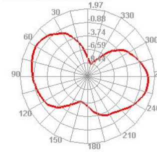
2500.000MHz E1
