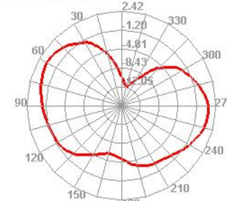
2450.000MHz E1
