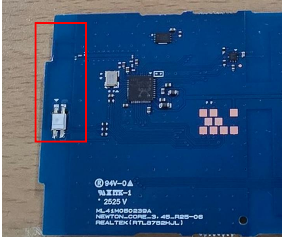
[NFC Antenna(RX)]
