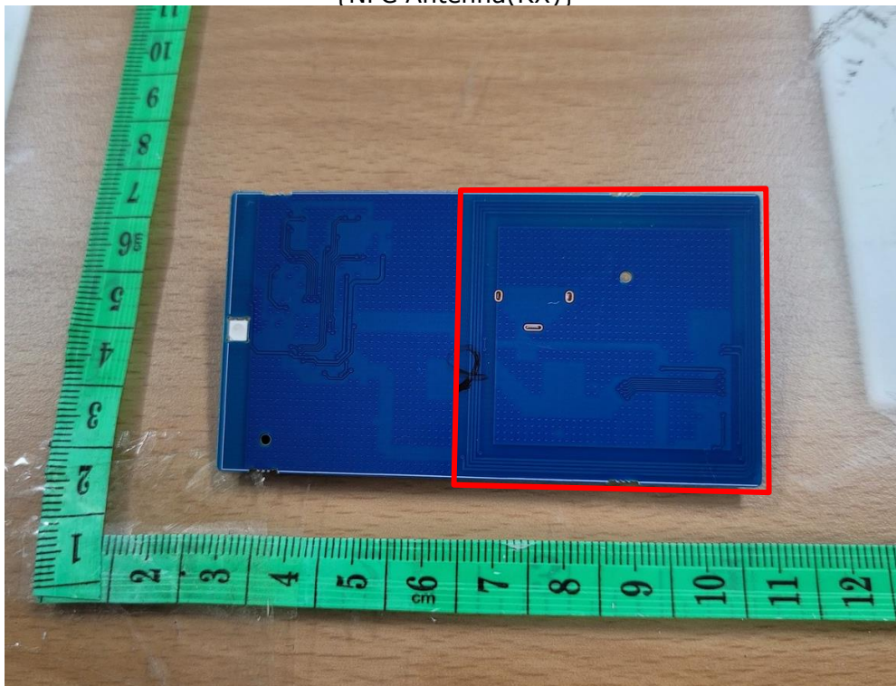
{NFC Antenna(RX)}
