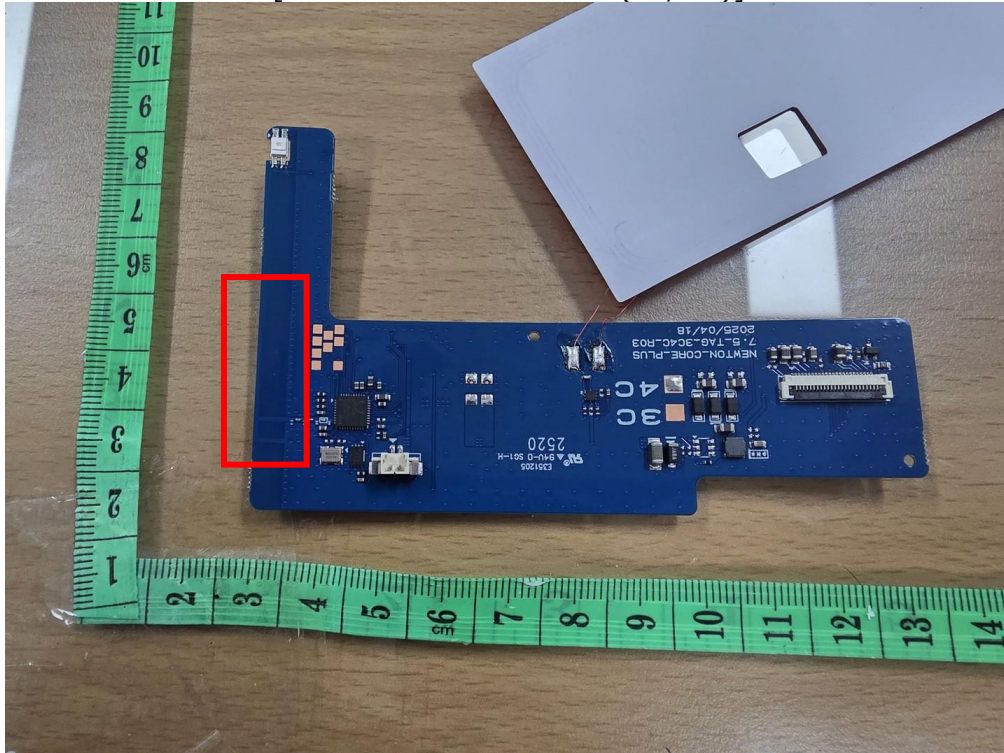
[NFC Antenna(RX)]
